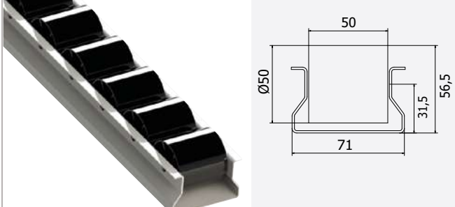
CVRT-18 - PP Makara
