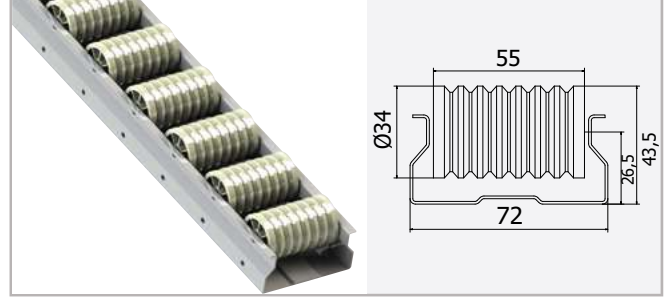
CVRT-11 - Elastomer Makara, Yüzeği Tırtıllı
