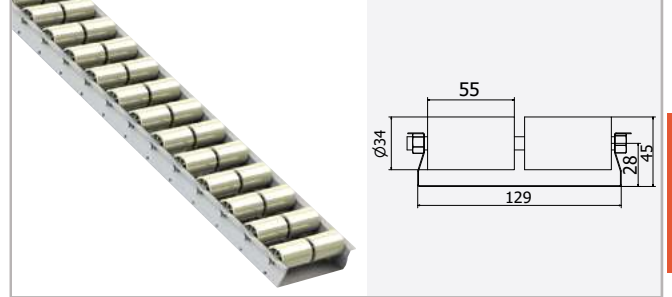
CVRT-13 - Elastomer Makara, Yüzeği Düz
