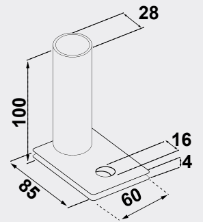
CV-CT44 (CV-CT02 için Soket Takımı)
