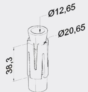
CV-CT44 (CV-CT02 için Soket Takımı)
