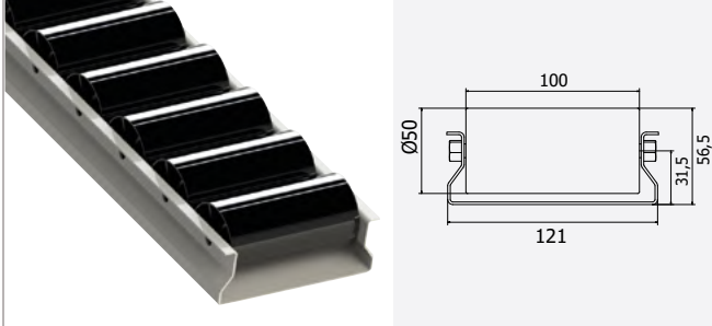
CVRT-16 - PP Makara
