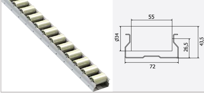
CVRT-10 - Elastomer Makara, Yüzeği Düz
