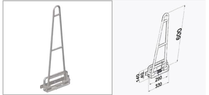
CV-TTF03B / AĞIR TİP
