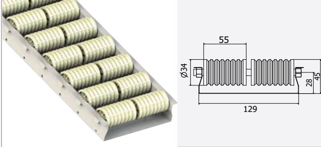
CVRT-14 - Elastomer Makara, Yüzeği Tırtıllı
